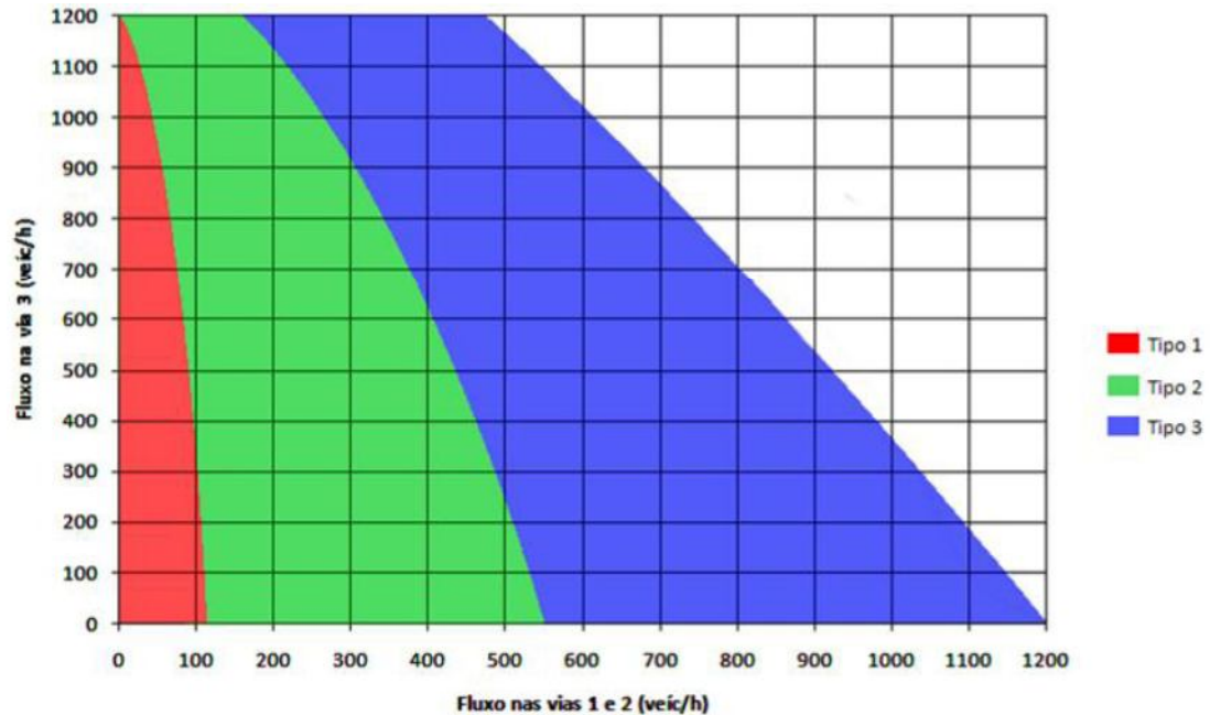
Figura 12: Operação mais eficiente em função dos fluxos
