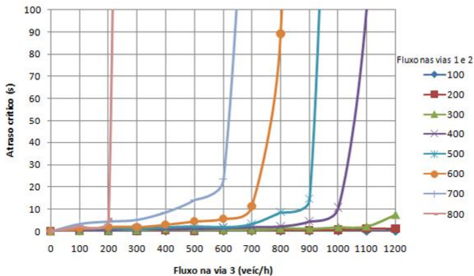
Figura 9: Atraso X Fluxo – Rotatória com preferencial para as vias 1 e 2
