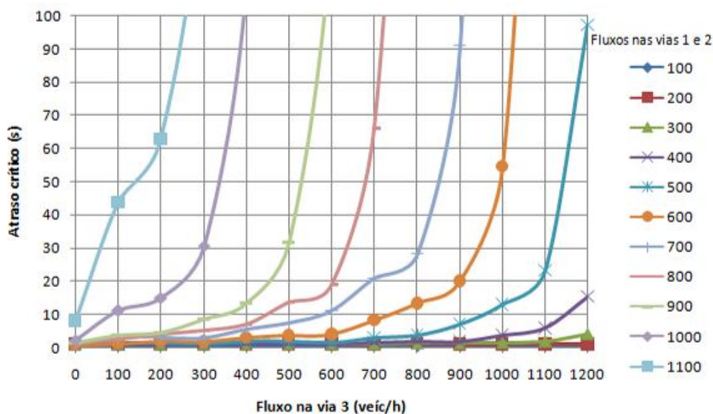
Figura 11: Atraso X Fluxo – Rotatória com formação de pelotão
