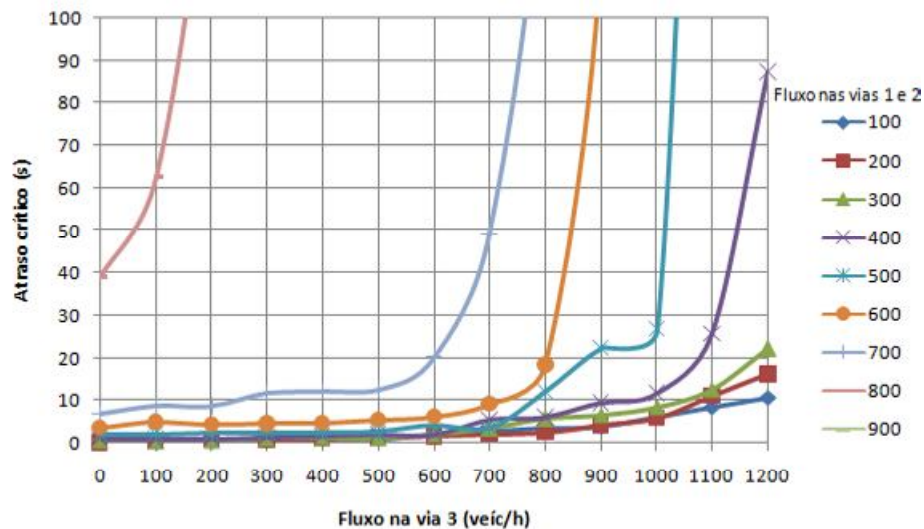
Figura 8: Atraso X Fluxo – Rotatória com preferencial para veículos circulantes
