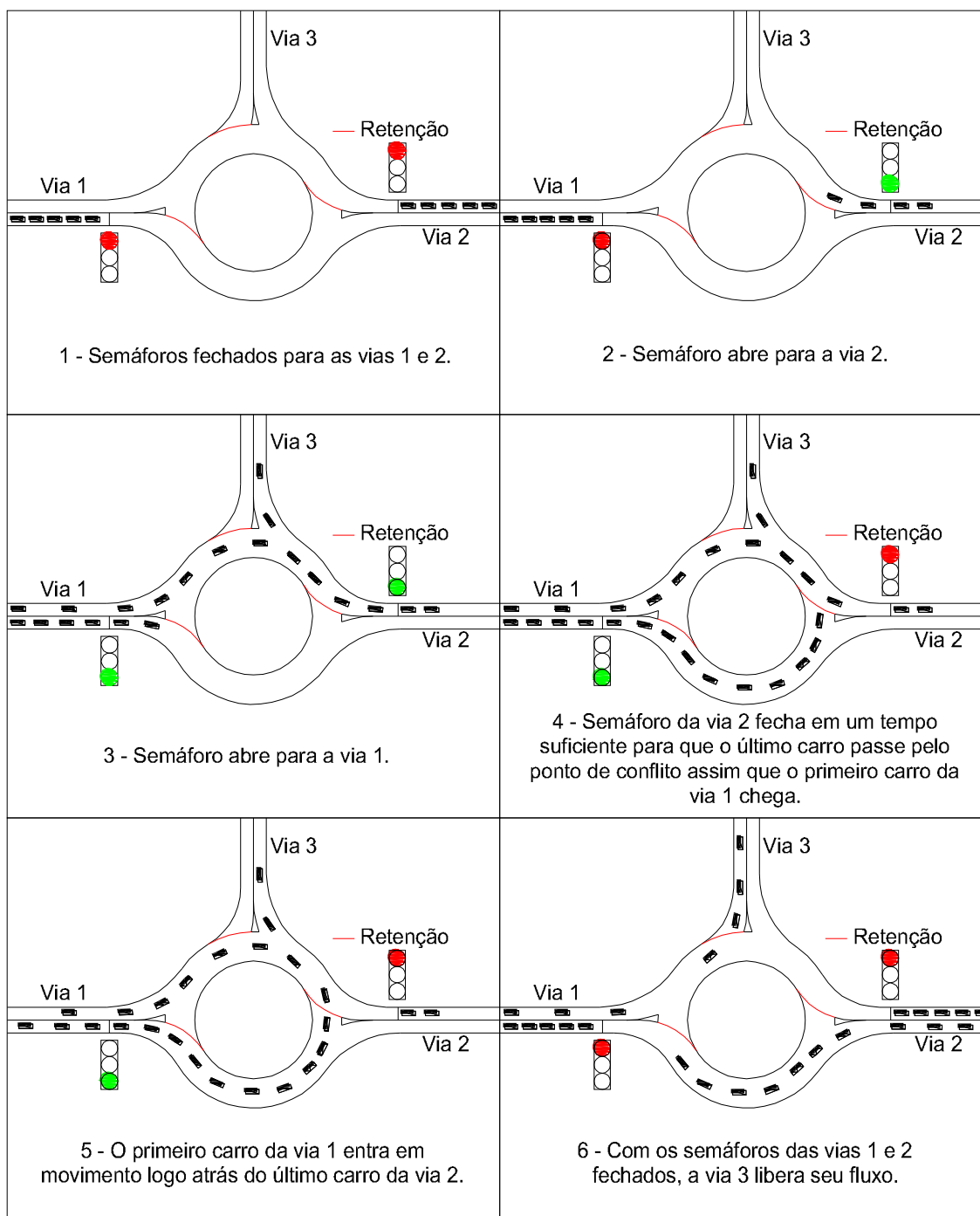
Figura 7: Esquema de operação da rotatória com formação de pelotões
