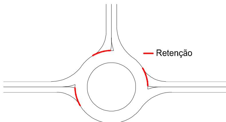
Figura 3: Rotatória com prioridade para a via circular
