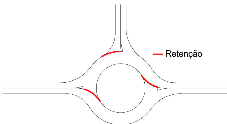
Figura 4: Rotatória com prioridade para a via principal
