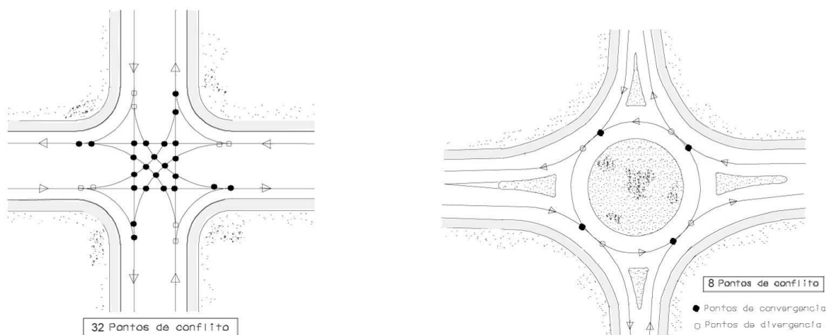
Figura 1: Pontos de conflitos
