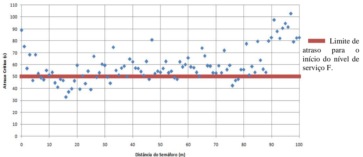
Figura 6: Variação no atraso crítico em função da distância dos semáforos
